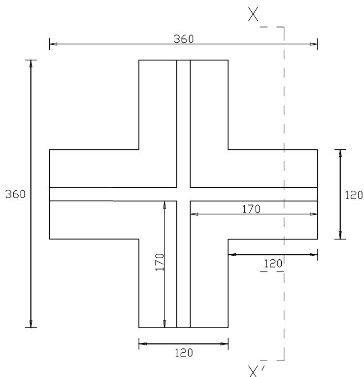
PIANTA/FRONTE
