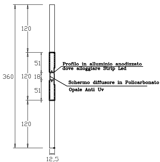
SEZIONE X-X'
