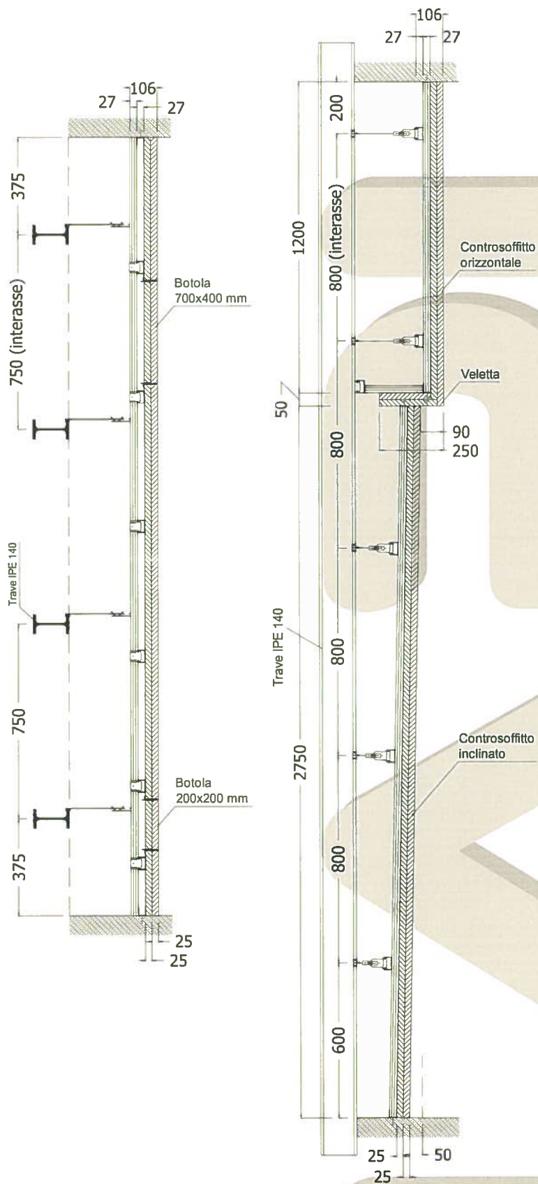
Particolare sezione
