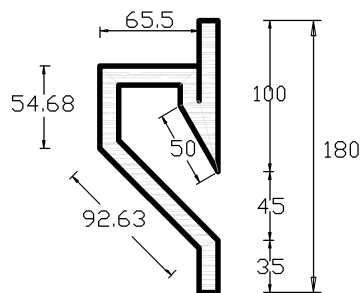
SEZIONE X-X'
