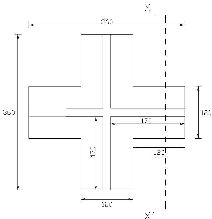
PIANTA/FRONTI
