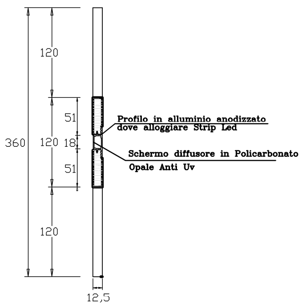
SEZIONE X-X'
