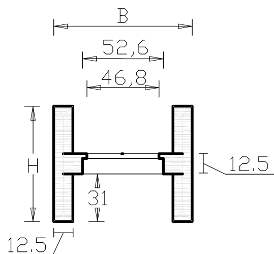
SEZIONE X-X\'
